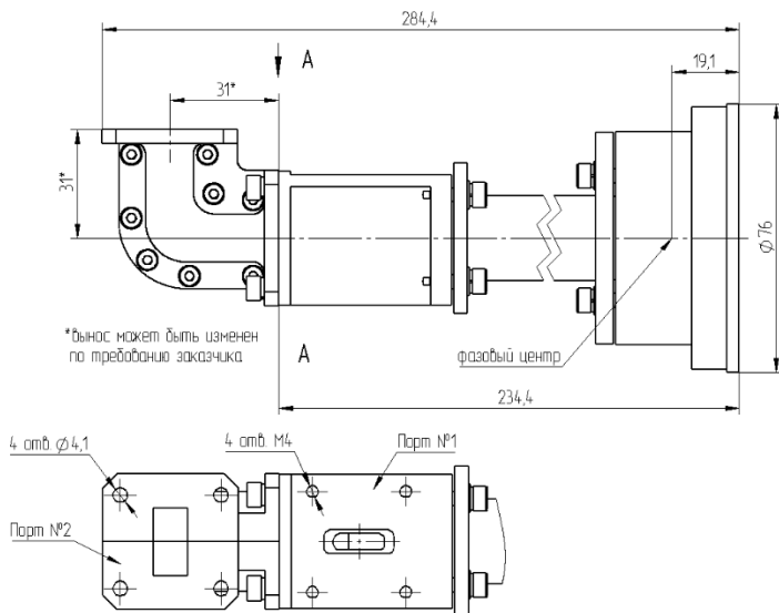
Рисунок 1 – Общий вид и габариты изделия.
